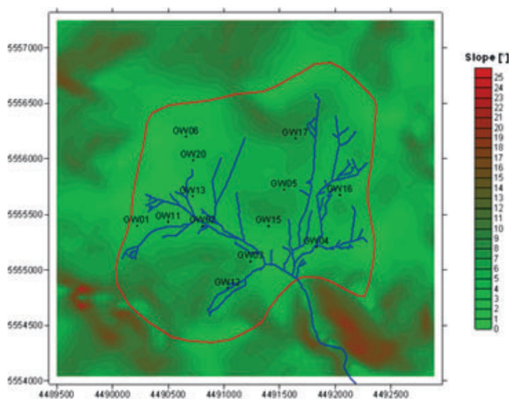
Abbildung 2: Grenzen eines kleinen hydrologischen Einzugsgebiets im Fichtelgebirge. Die Farben geben die Hangneigungen wieder. An den eingezeichneten Punkten befinden sich Grundwassermessstellen. (Quelle: G. Lischoid)
